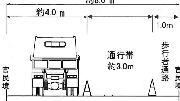
片側交互通行規制イメージ図
